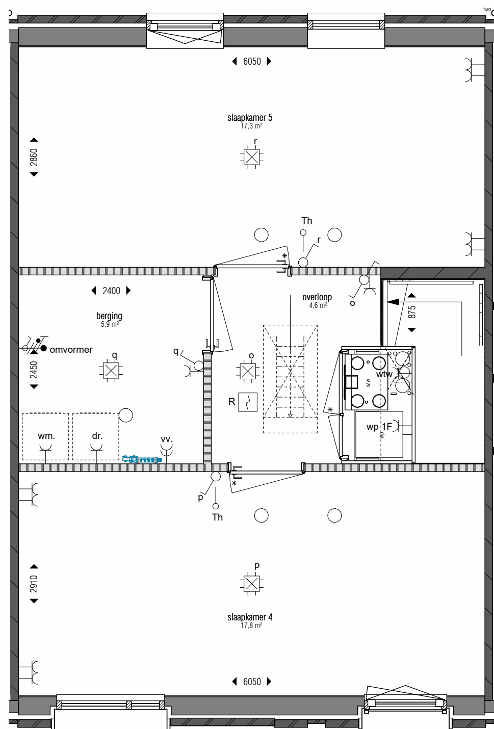
tweede verdieping 1 : 50
