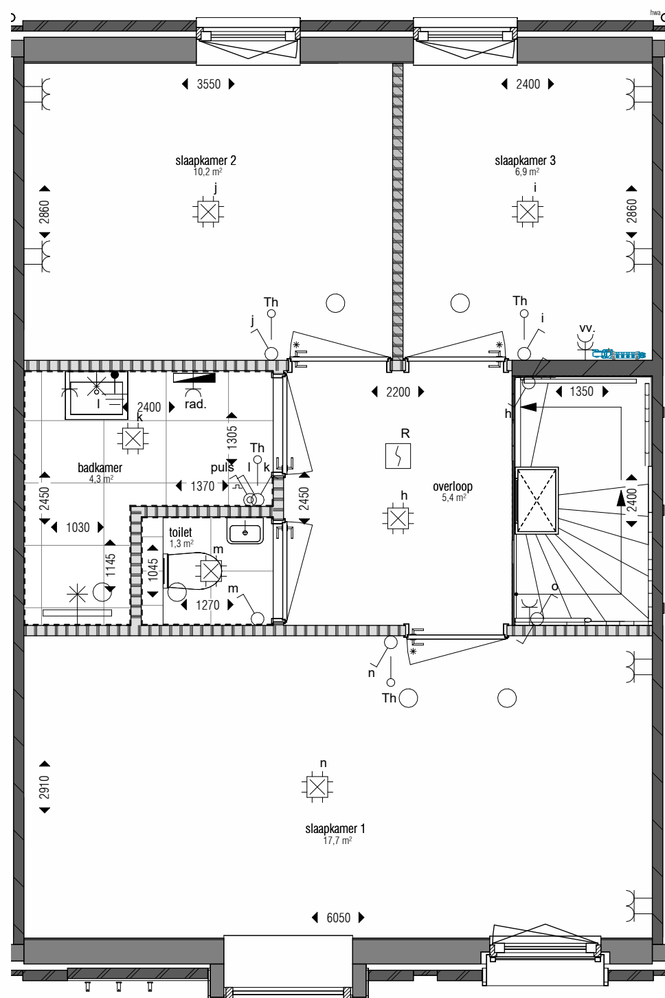
eerste verdieping 1 : 50
