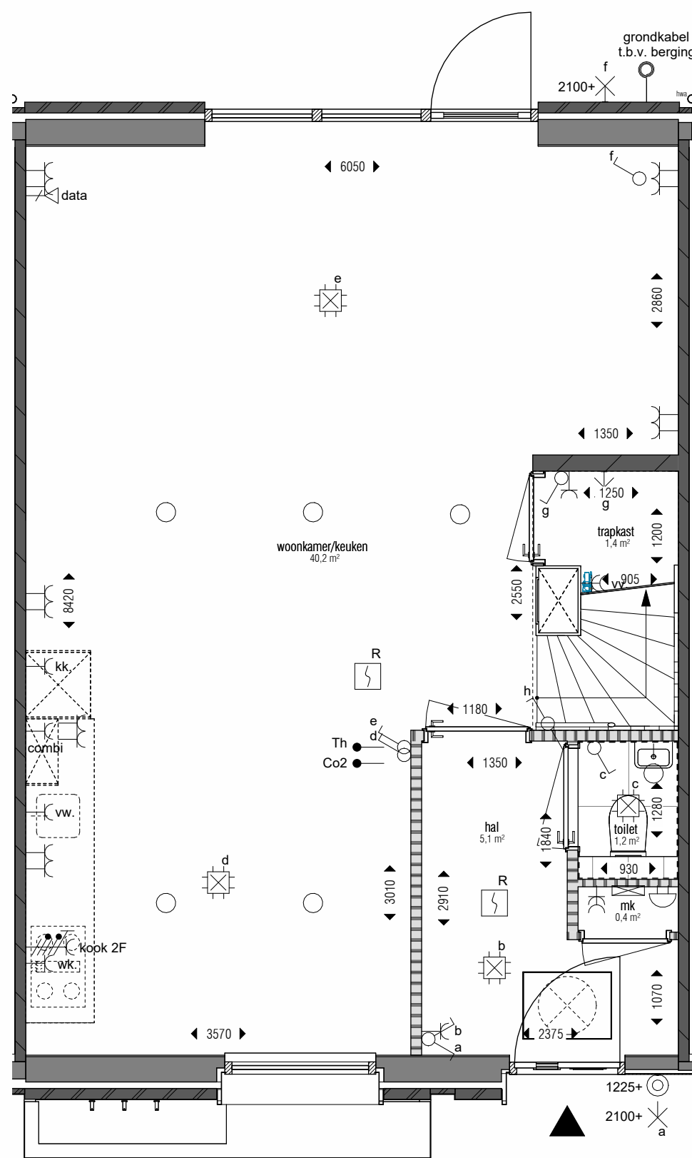
begane grond 1 : 50
